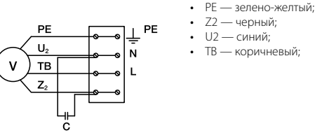
Схема 1 (230 В, 1 ф.)
